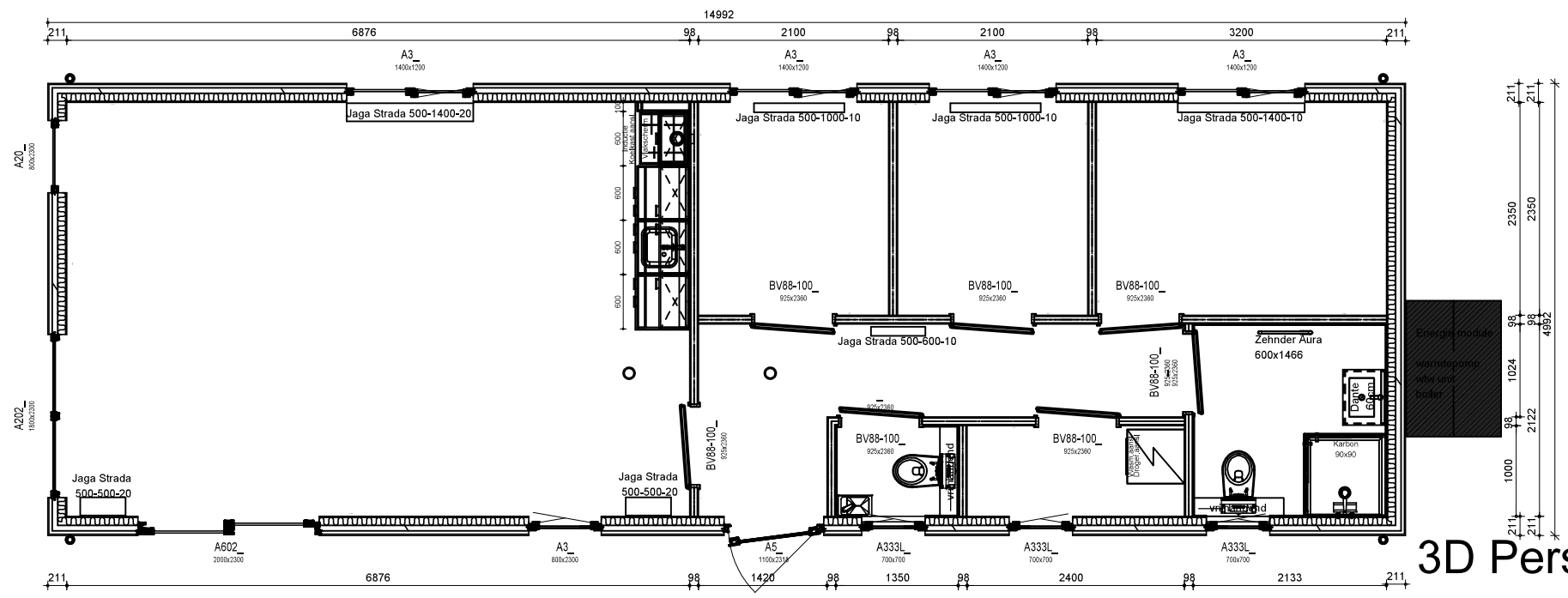
Plattegrond
